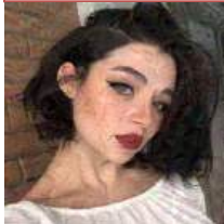
iFGSM ( \epsilon=0.1 )
